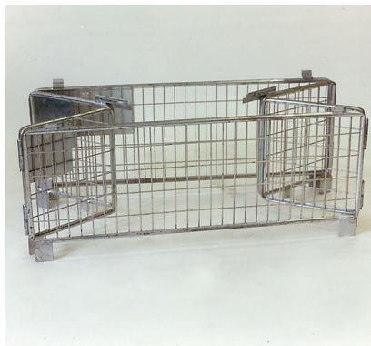
Normgitter 2525 RM beim Zusammenklappen Cadre grillagé normalisé 2525 RM au pilage
